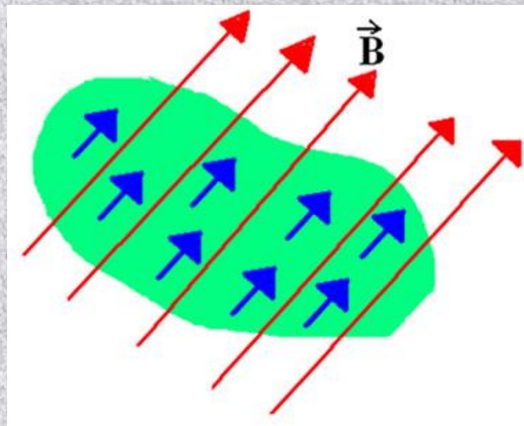
Erős mágnes közelében a részecskék iránya megváltozik
